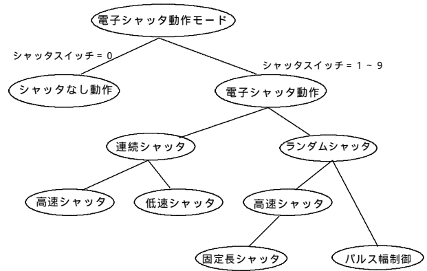
図 5 - 1 電子シャッタ動作モード
