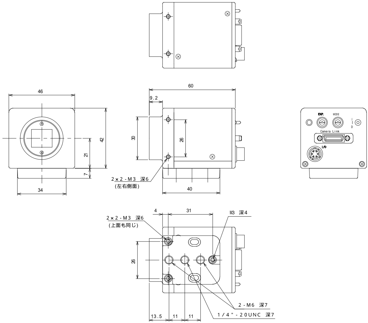
图 1 1 - 1 FC5100SPL外形图
