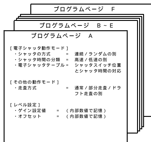
図 5-2 プログラムページ の概念図
