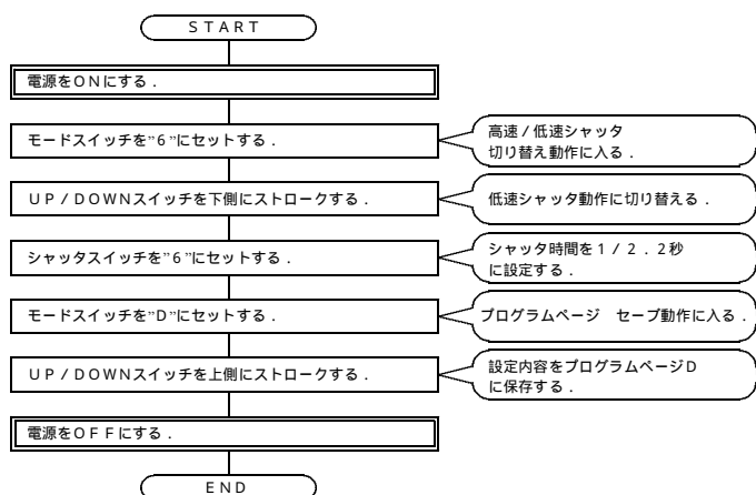
図 6 - 5 連続 / 低速シャッター動作 (1/2.2秒) で使用する手順例 1
