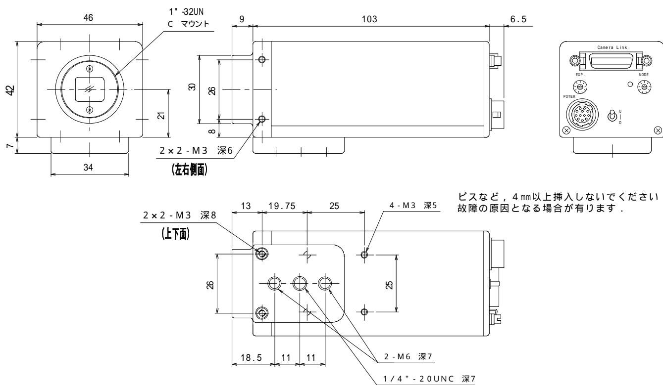
図 1.1 - 1 FC2000CL外形図
