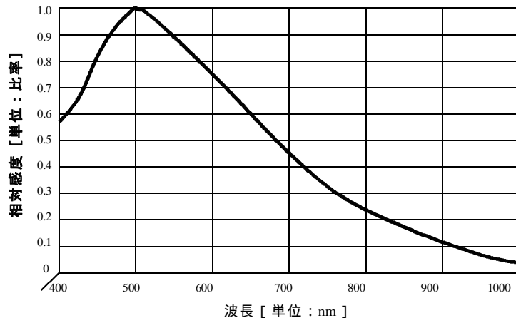
FC2000CLの代表的感度特性例
