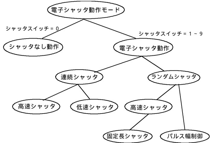
図5 - 1 電子シャッター動作モード
