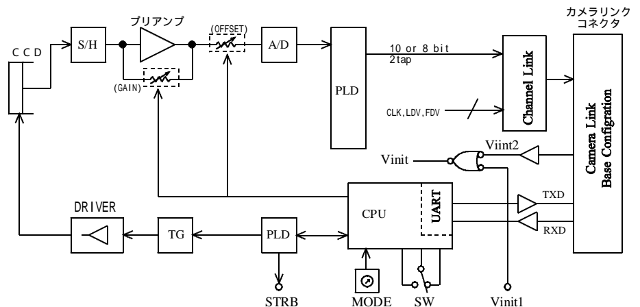
本機のブロック図
