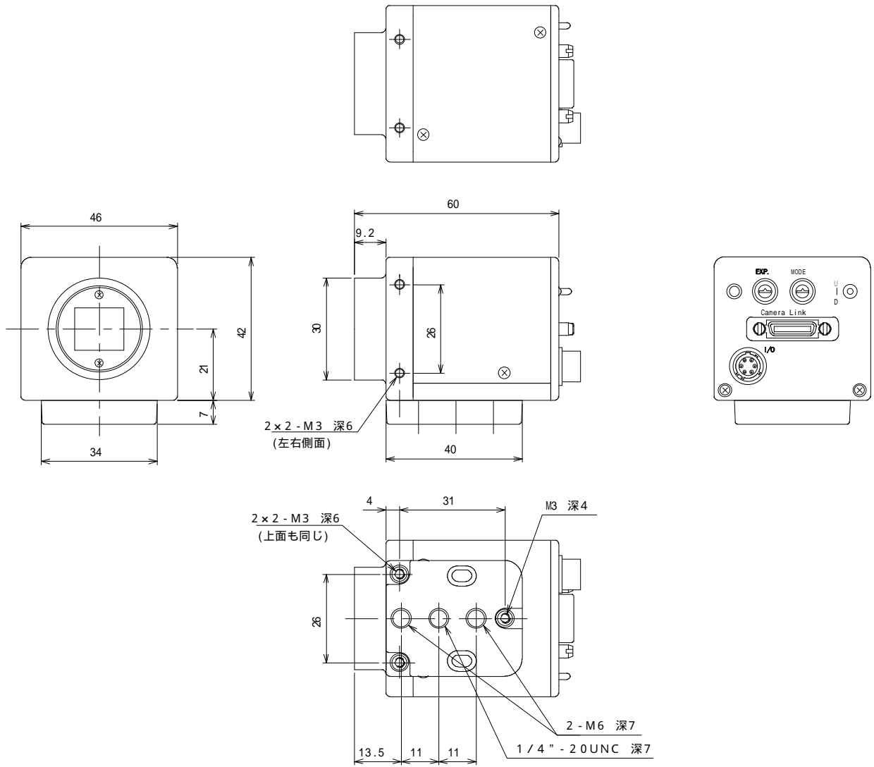
图 1 1 - 1 FS5100SPL外形图
