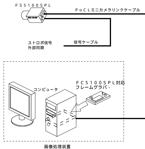
図 4 - 1 カメラと周辺機器の接続例
