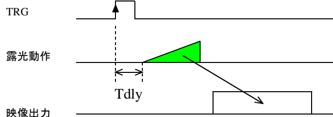
図 4-5 トリガ信号の遅延
