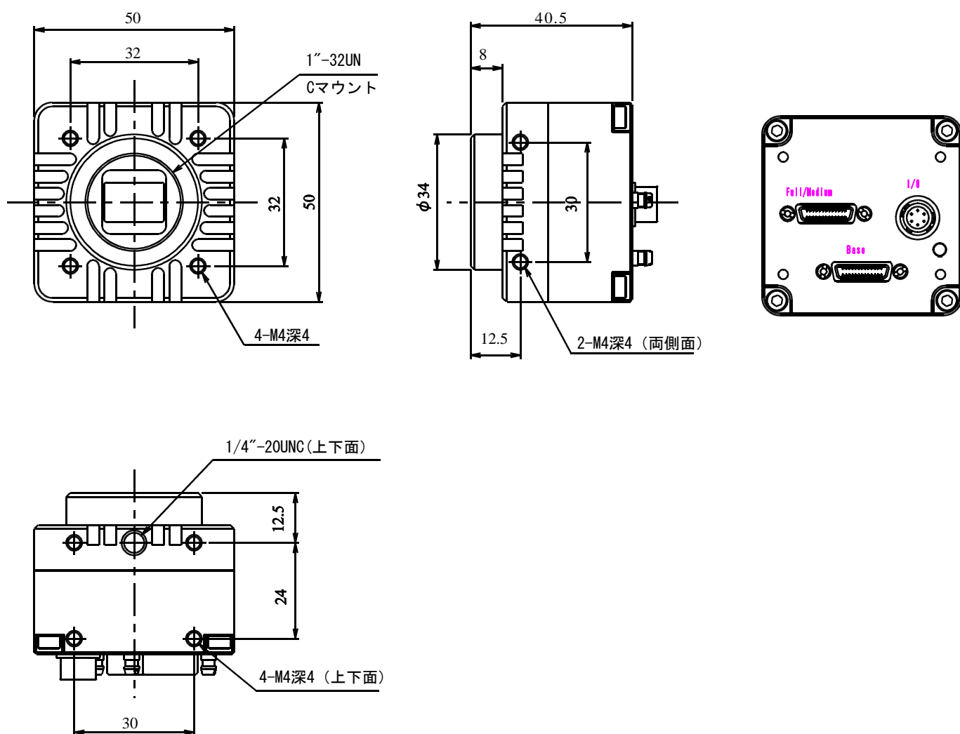
図9-1 FCM4MPL/FSM4MPL外形図
