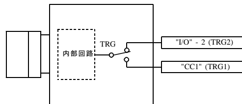
図 4-4 TRG 信号の内部接続
